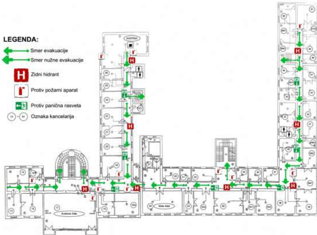
Слика 8: План евакуације спрата зграде општине Бечеј
