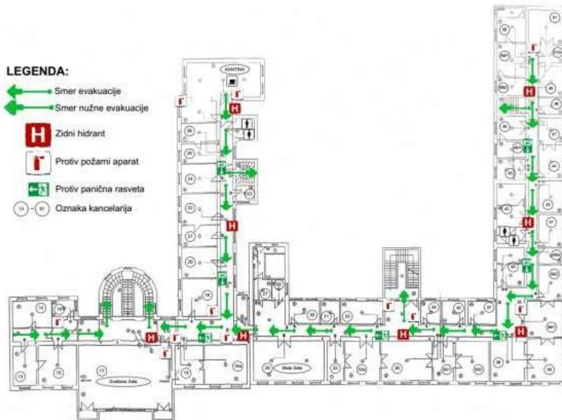
Слика 8: План евакуације спрата зграде општине Бечеј
